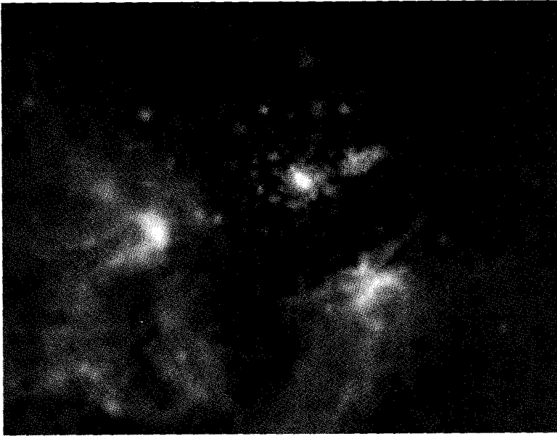
النجم بستول (الشمس) يقع على مسافة ٢ ألف ستة ضوئية حجمه يساوي ١٠ ملايين مرة حجم شمسنا يا سبحان الله
