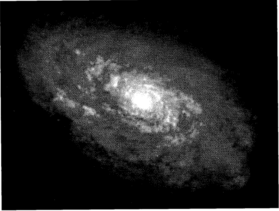
مجرة تتشكل من مجموعة هائلة من النجوم صورة من التلسكوب الأرضي الياباني وهي مجرة إهليلجية بيضاوية
