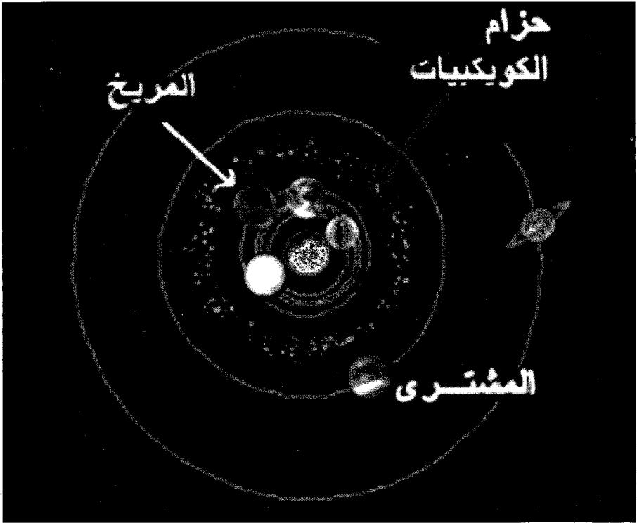
حزام الكويكبات يقع ما بين كوكب المريخ وكوكب المشتري
