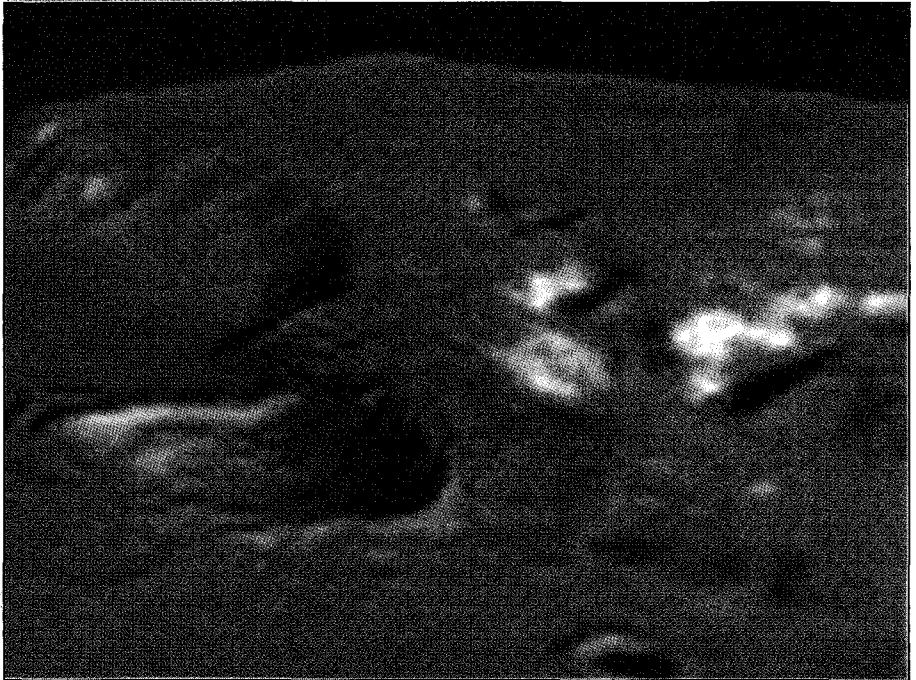
اكتشافات جديدة ومستمرة على سطح المريخ ويأمل العلماء بوجود حياة على هذا الكوكب
