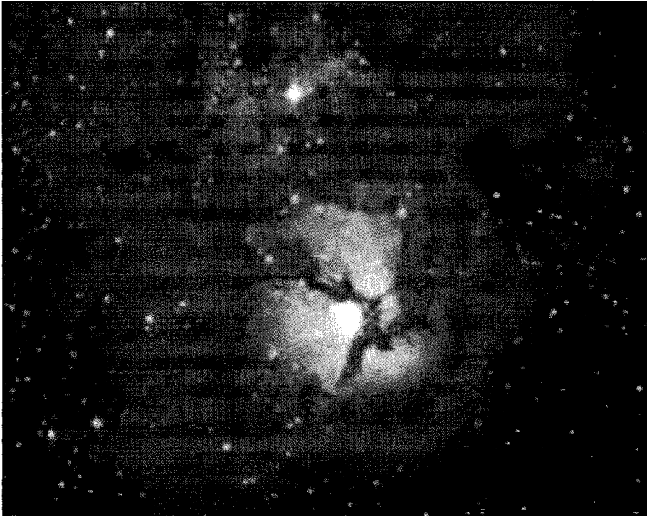
من مكتشفات هابل سديم ثلاثي الفصوص - منطقة ينكتل فيها الغاز والغبار معاً ليشكل النجوم الوليدة
