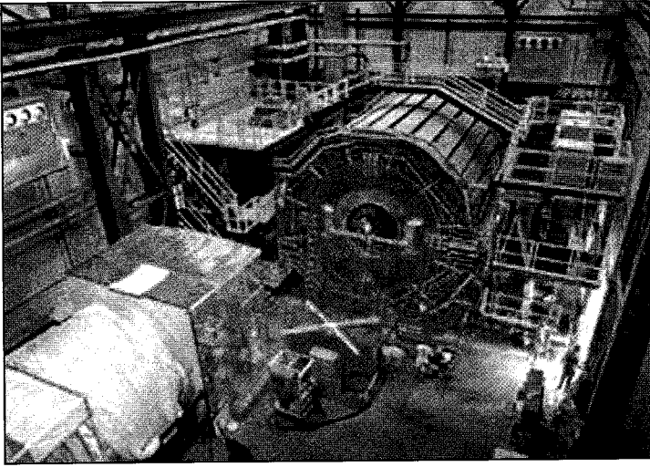
تجربة محاكاة الانفجار الكبير ونشأة الكون والثقوب السوداء في المختبر
