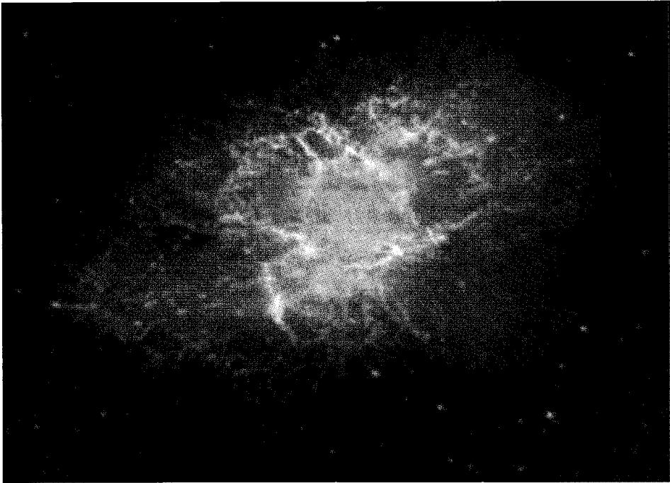
نجم نيوتروني في سديم السرطان يدور على محوره ٣٠ مرة في الثانية يرسل أشعة سينية من مركز السديم
