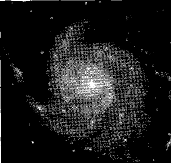
مجرة لولبية - حلزونية
