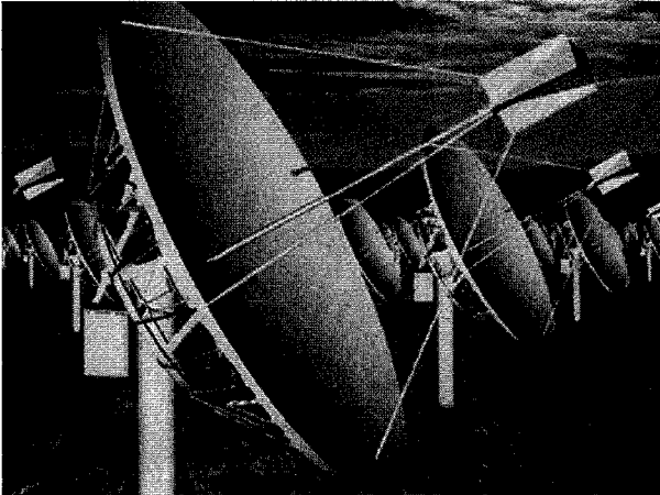
تلسكوب منظومة ألن أضخم تلسكوب في التاريخ البشري صور تطور صناعة التلسكوبات وتصور عدد التلسكوبات المربوطة مع بعضها فتؤلف هذه المنظومة
