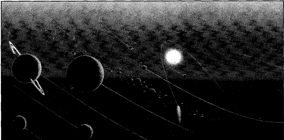
صورة تبين الكواكب القريبة من الشمس وهي عطارد - الزهرة - الأرض - المريخ - المشتري
