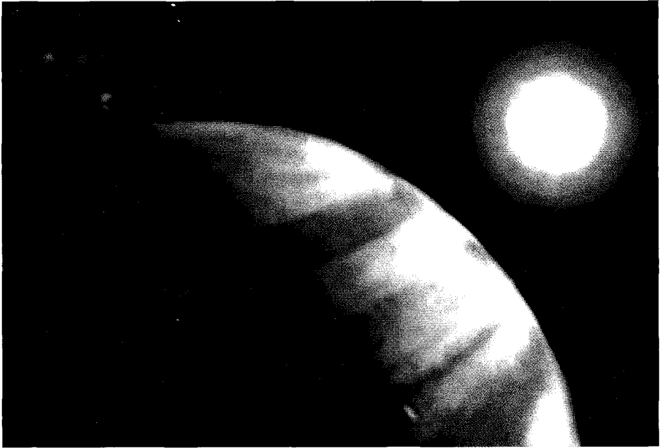
كوكب نبتون تم اكتشافه عام ١٨٤٥ وهو أحد كواكب المجموعة الشمسية وفي الصورة ثلاثة أقمار تم اكتشافها حديثاً
