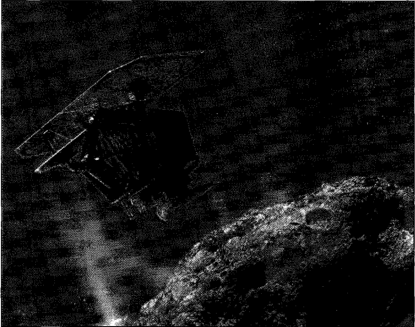
مركبة ديب أمباكت قرب مذنب تيمبل قبل الإصطدام بعد أن انفصلت عن العربة الأم
